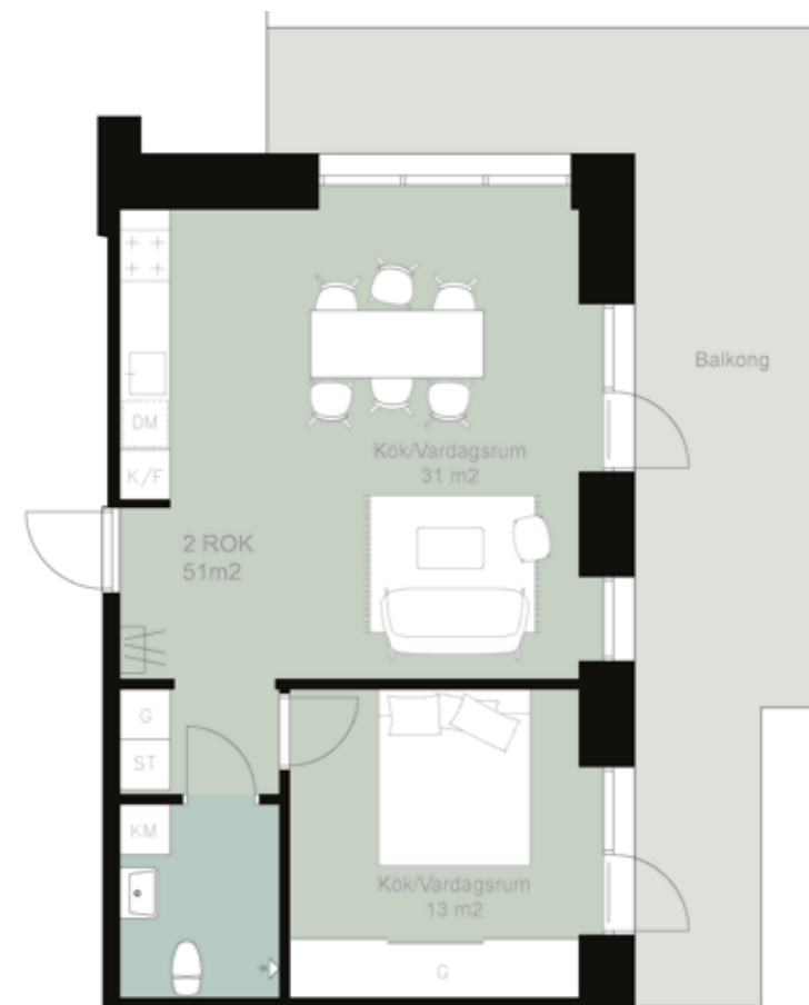
Lägenhet 6-1302, 6-1304 7-1302, 7-1304 8-1302, 8-1304
